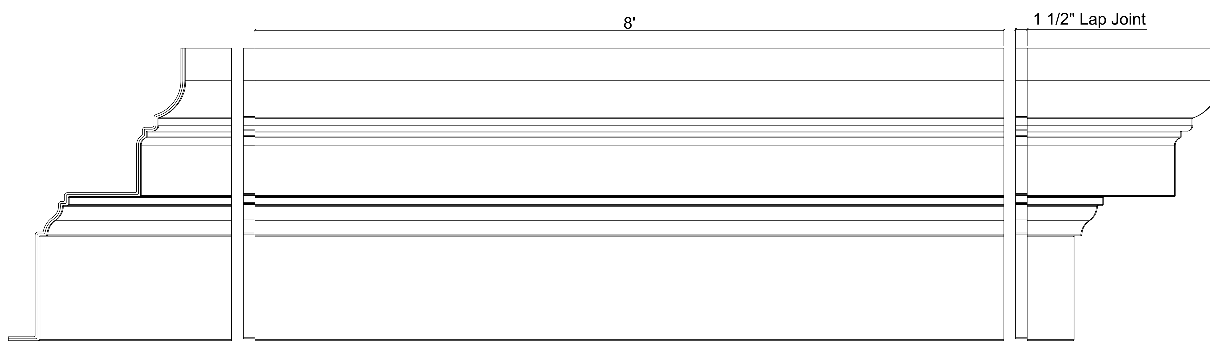
5 CR226x8 Elevation SCALE 1:1
